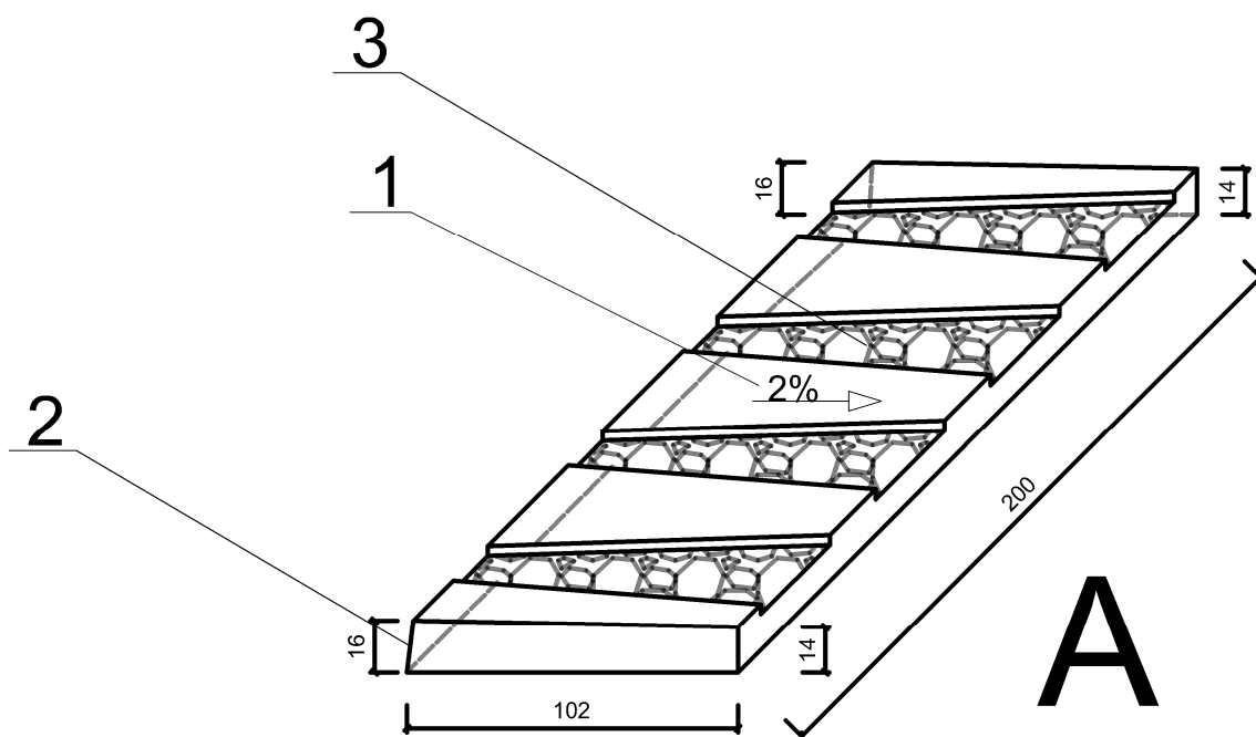
rys. 2 Schemat systemu powierzchniowego odwodnienia płyty betonowej prefabrykowanej
