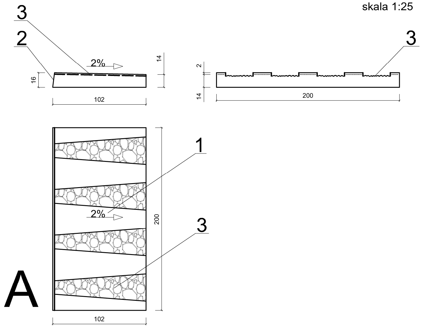
rys. 1 Schemat drogowej płyty betonowej ze spadkiem
