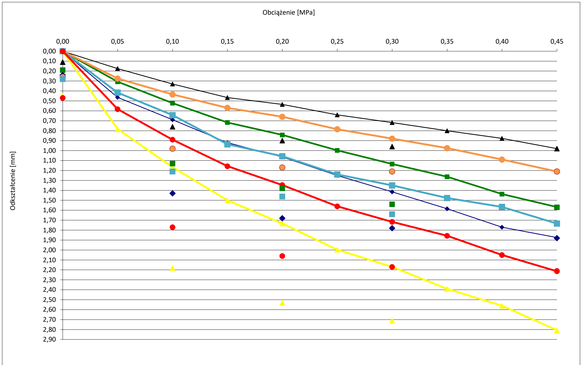
Wykres ugięć wtórnych obciążenie i odciążenie dla różnych nawierzchni
